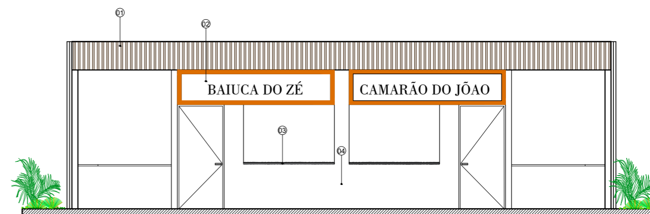
VISTA B ESC. 1/75
