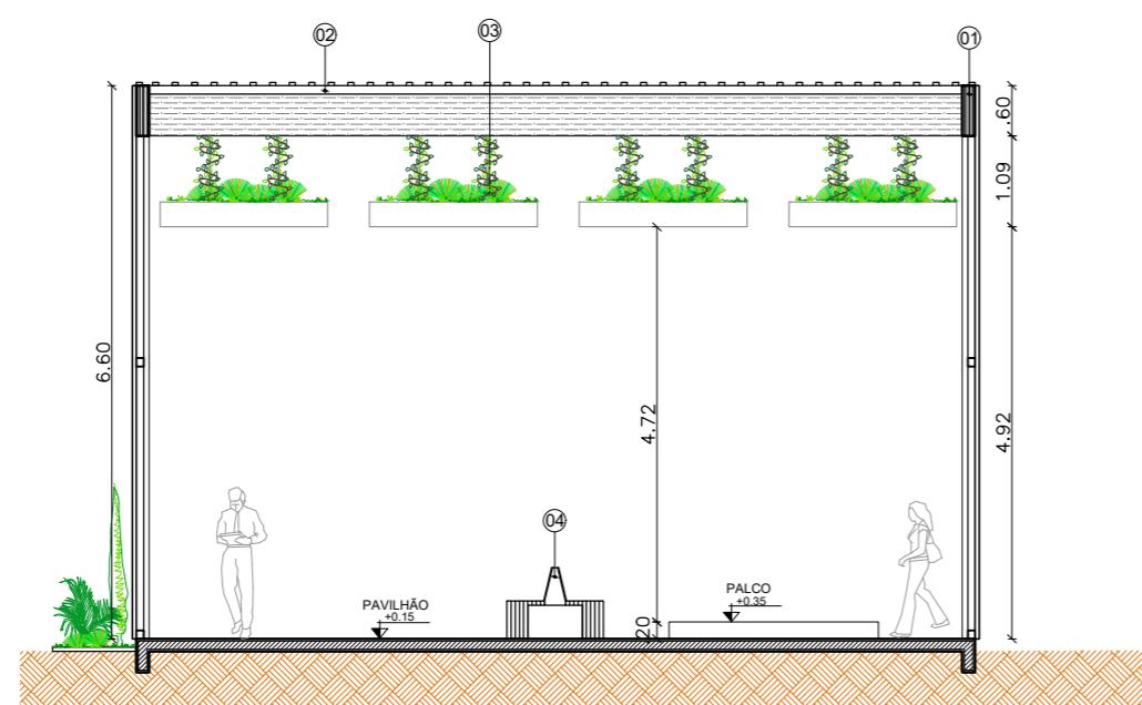
CORTE BB' ESC. 1/100
