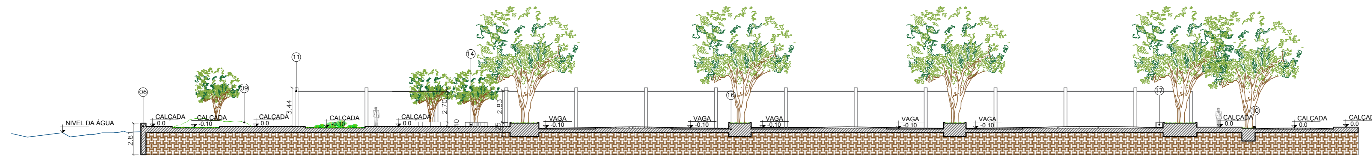
CORTE DD ESC.1/200
